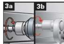
3a 3b Draai de betonschroef vast met een steeksleutel (sleutelmaat SW 15). Neem de maximale aandraaimomenten in acht.
